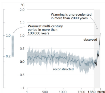
Historique des températures, la célèbre crosse de hockey
